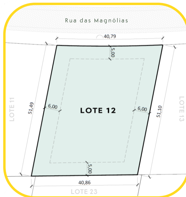
PLANTA DO LOTE
