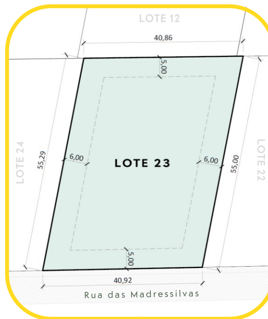
PLANTA DO LOTE
