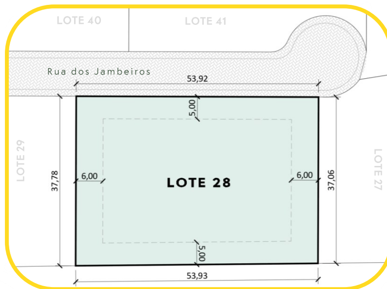
PLANTA DO LOTE
