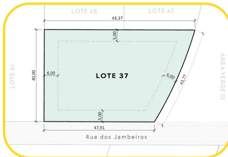
PLANTA DO LOTE
